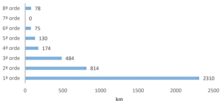
Figura 1: Comprimentos totais das linhas de água segundo a classificação Strahler (1957) na bacia internacional do rio Minho
